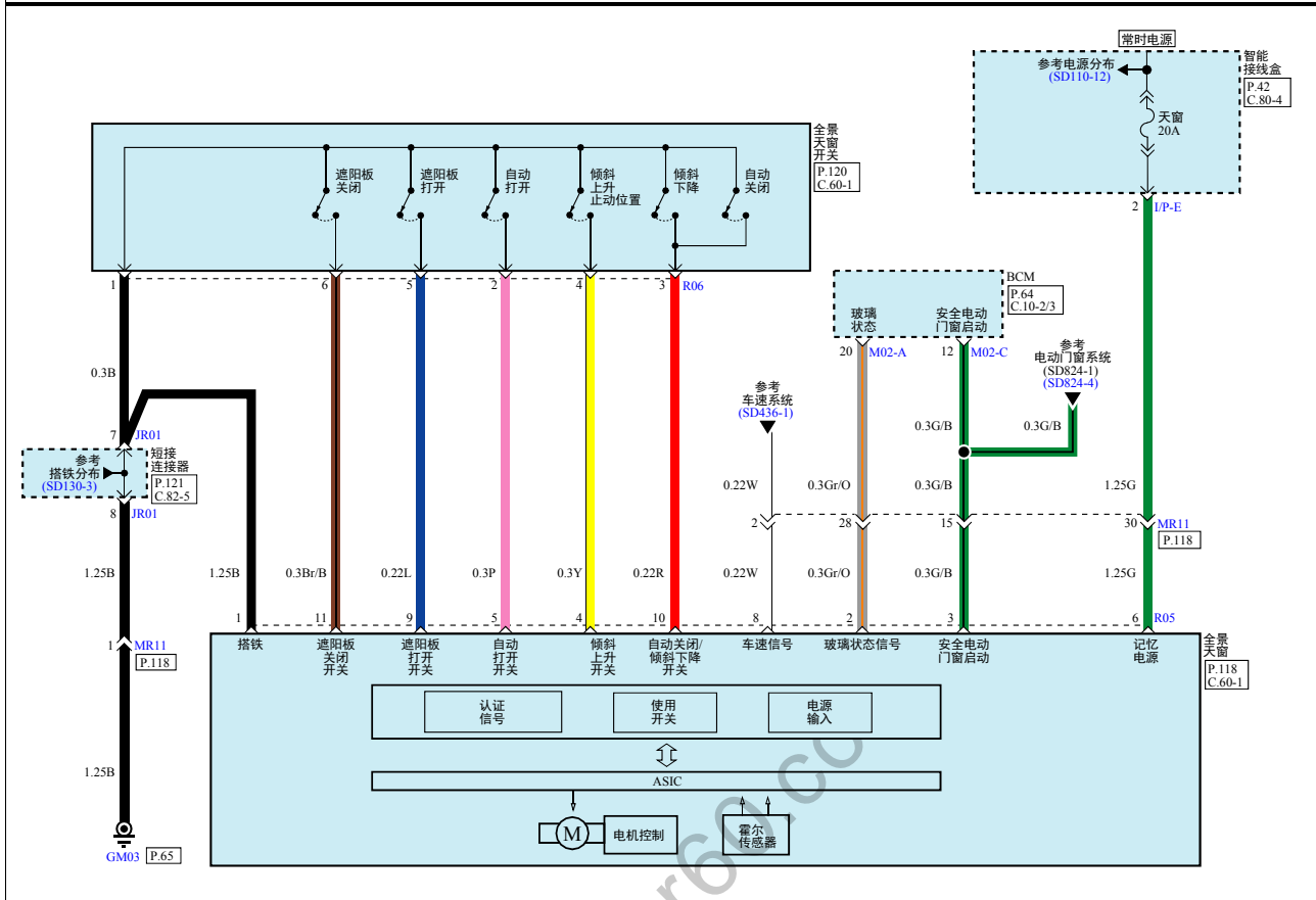
天窗系统(1)
